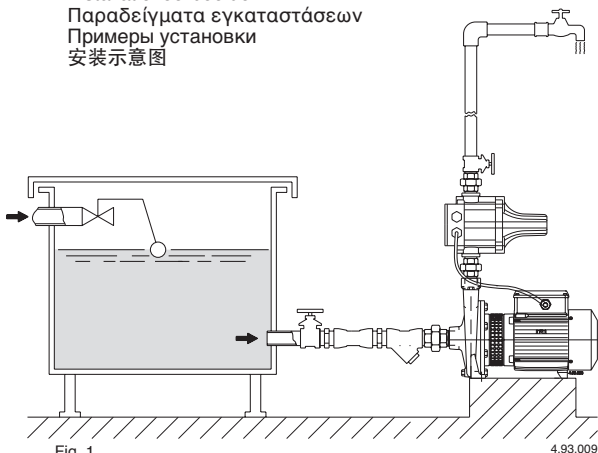
Fig. 1 Funzionamento sotto battente Positive suction head operation Zulaufbetrieb Fonctionnement en charge Funcionamiento bajo carga 正吸水头的操作
